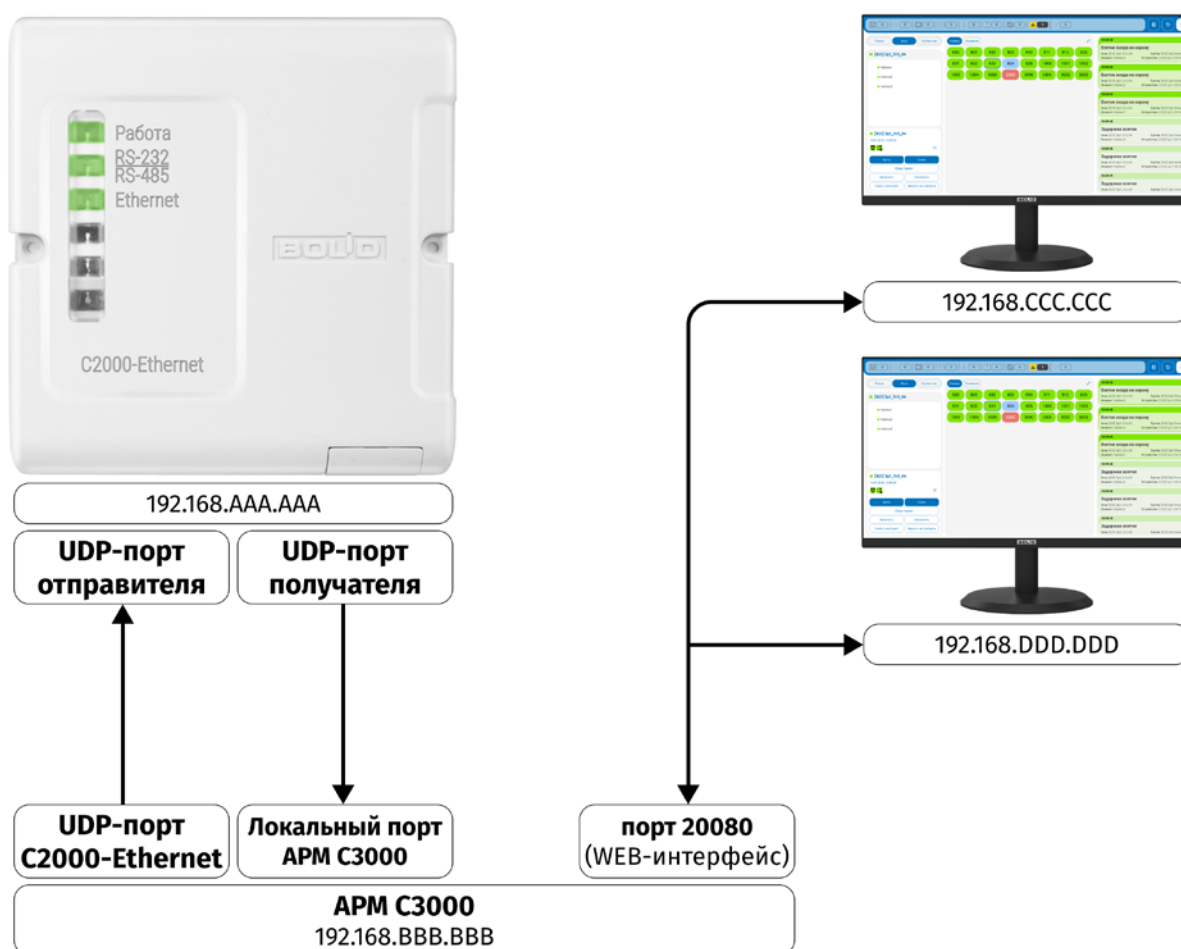
Рисунок 2. Общая схема соответствия параметров конфигураций «C2000-Ethernet» и АРМ «С3000»
