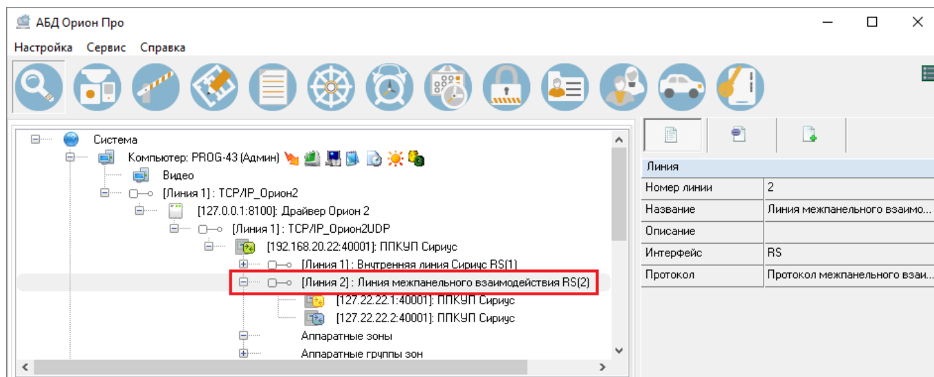
Рисунок 6-127 Линия межпанельного взаимодействия ППКУП "Сириус"
