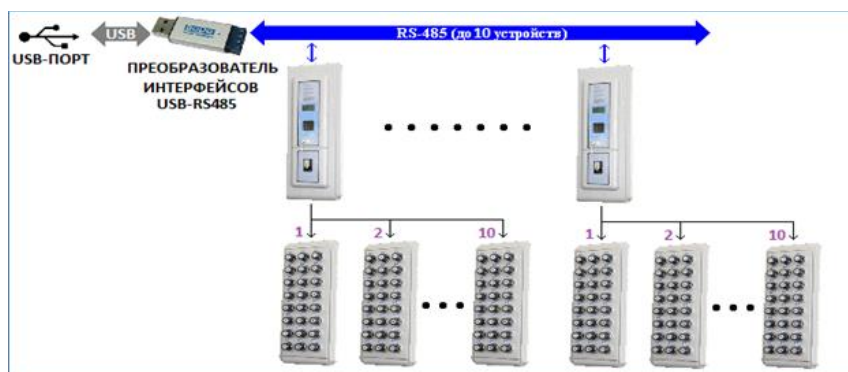
Рисунок 1-16 Схема подключения электронных сейфов для ключей к USB-порту
