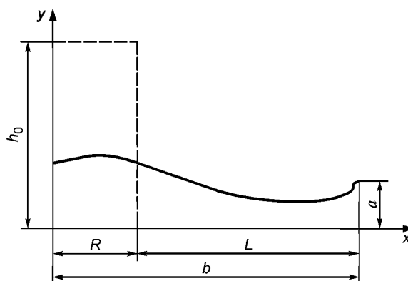
Рисунок К.2 — Типичная картина движения жидкости в обваловании при мгновенном разрушении резервуара
