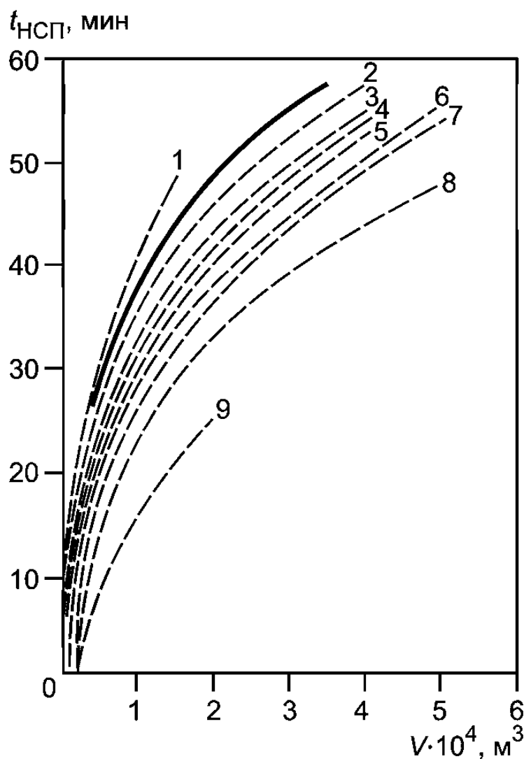
Рисунок Р.1 — Зависимость минимальной продолжительности начальной стадии пожара ( t_{\text{нсп}} ) от объема V , высоты H помещения и количества горючей нагрузки q , приведенной к древесине.
