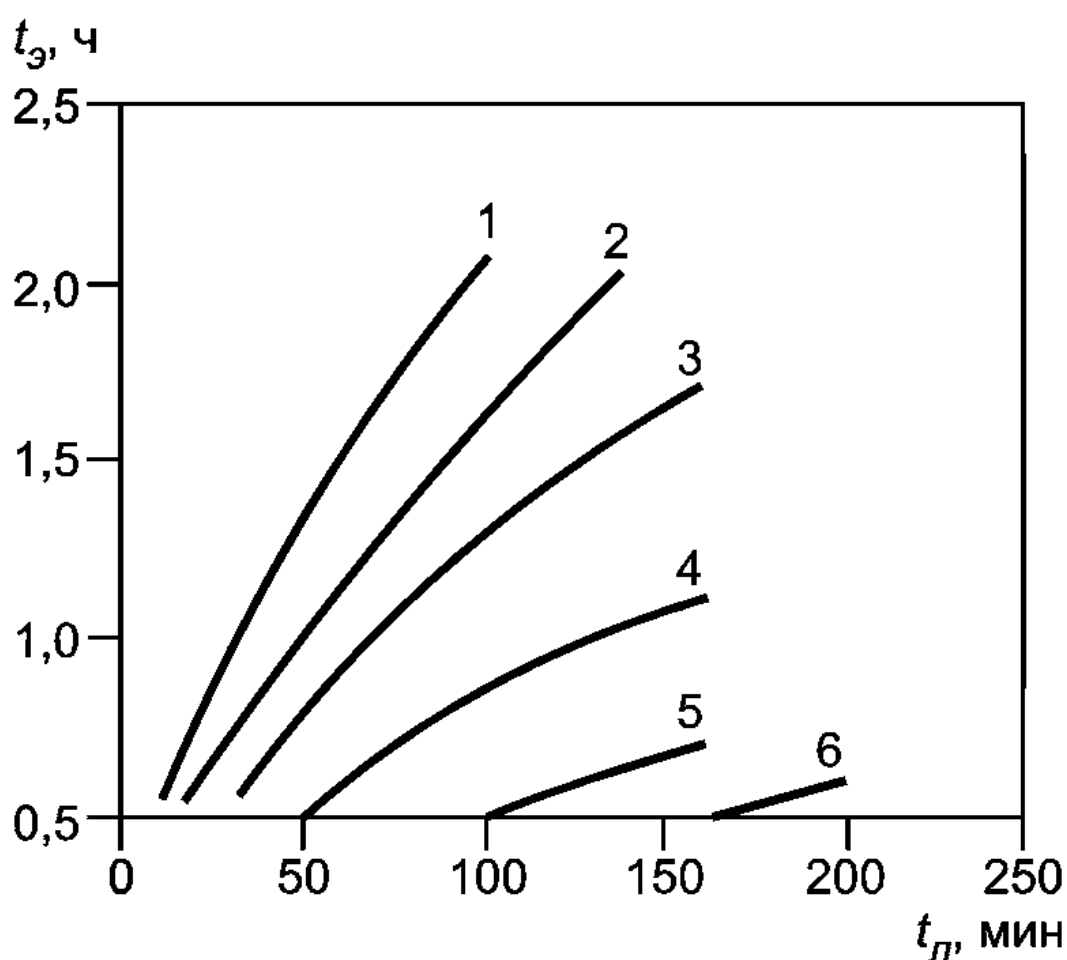
Рисунок Р.4 — Зависимость эквивалентной продолжительности пожара t_3 от продолжительности пожара t_d для железобетонных и огнезащищенных металлических конструкций перекрытия при горении ЛВЖ и ГЖ
