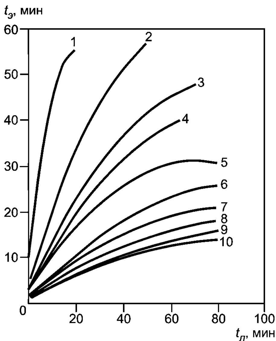
Рисунок Р.5 — Зависимость эквивалентной продолжительности пожара t_{\text{э}} от продолжительности пожара t_{\text{л}} для горизонтальных незащищенных металлических конструкций
