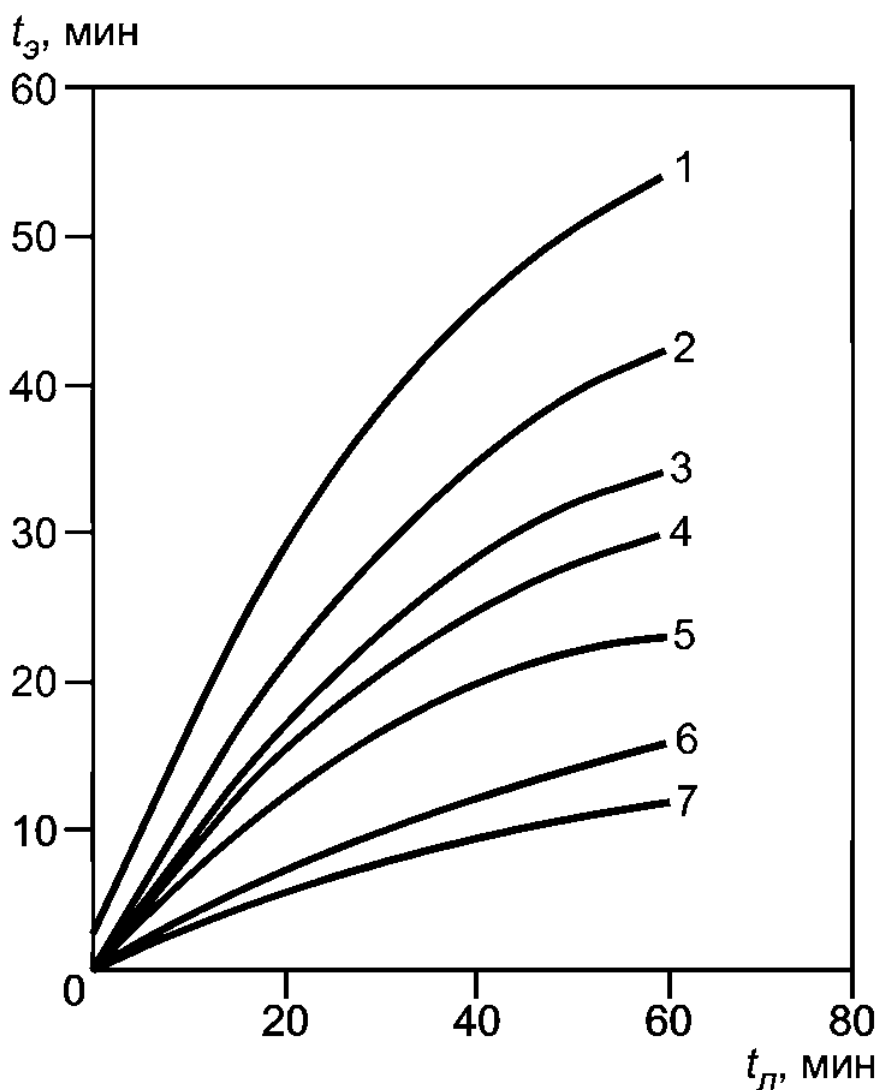
Рисунок Р.6 — Зависимость эквивалентной продолжительности пожара t_3 от продолжительности пожара t_d для вертикальных незащищенных металлических конструкций
