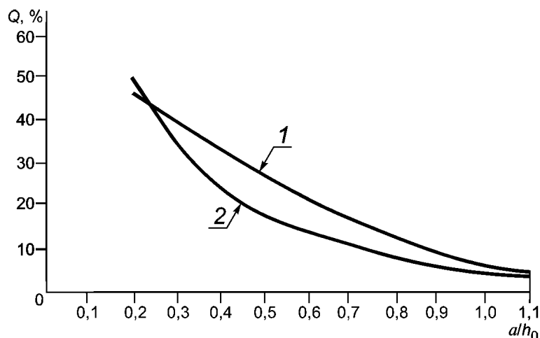
Рисунок К.3 — Зависимость доли перелившейся через обвалование жидкости Q от параметра alh_0 : 1 — расчет; 2 — эксперимент
