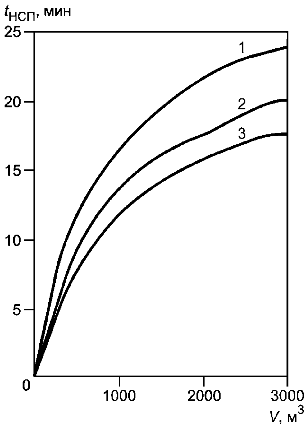
Рисунок Р.2 — Зависимость минимальной продолжительности начальной стадии пожара ( t_{НСП} ) от объема V и высоты H помещения
